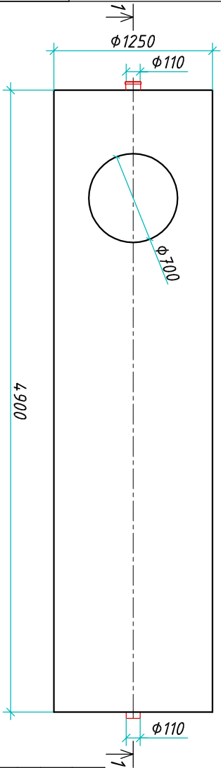
Вид сверху
